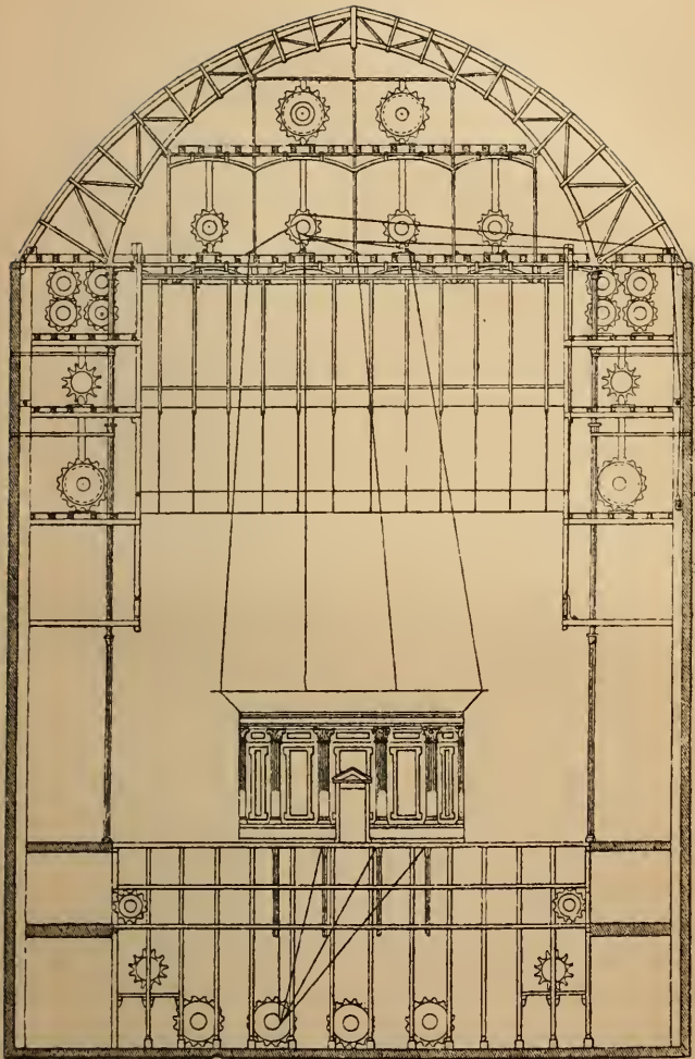
Fig. 61 — Coupe transversale. (Une ferme et un plafond équipés.)
